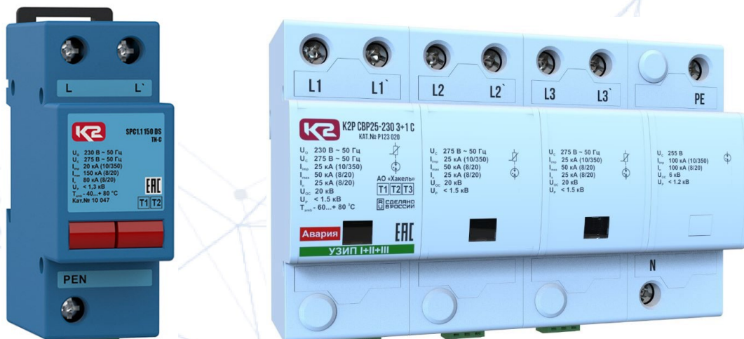
Рис.4 Маркировка устройств защиты от импульсных перенапряжений класса I+II серии SPC и класса I+II+III серии K2P CB (CBP). Информация пользователя.
