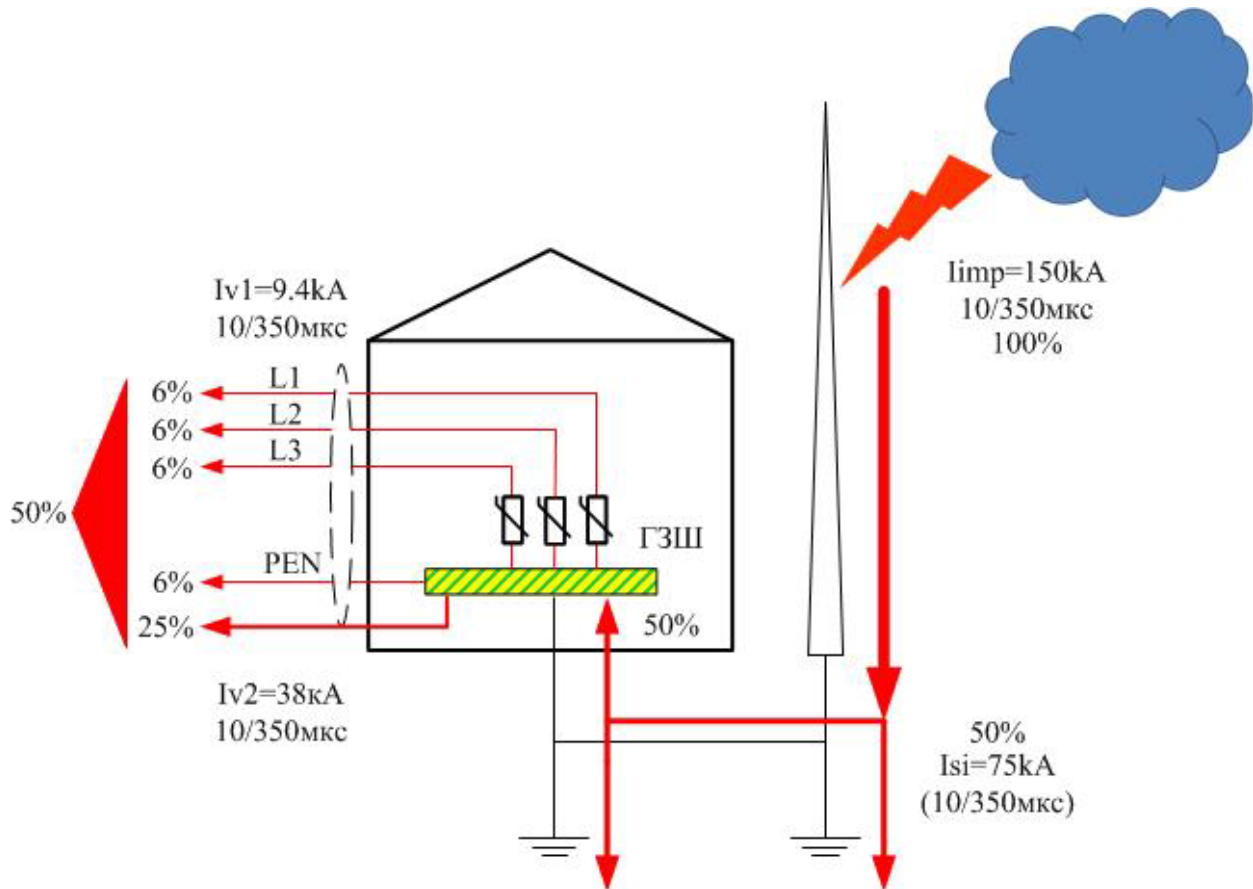
Рис.2. Оценка токов растекания
